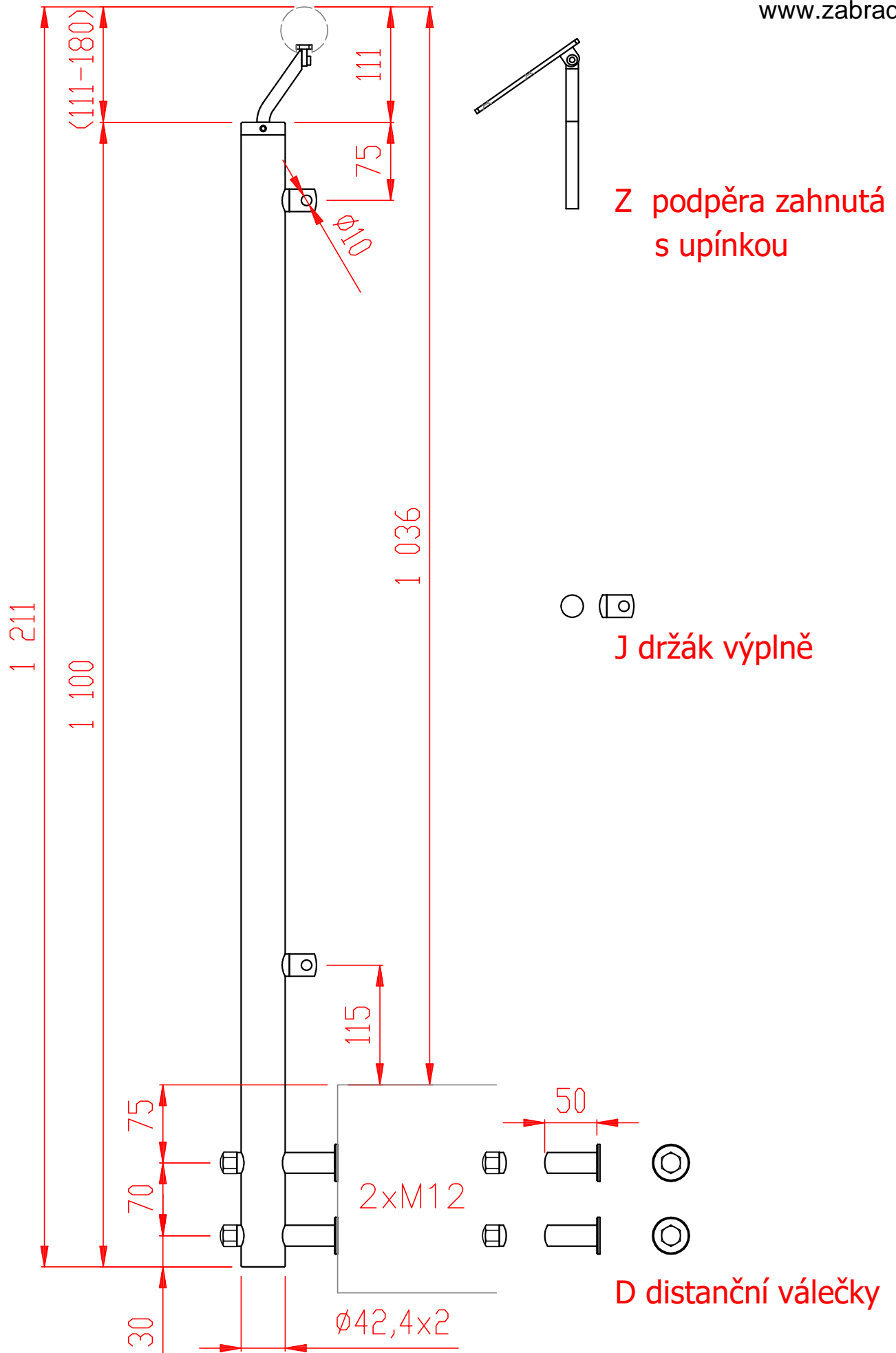
SL1270 - SMART svisle DZJ
